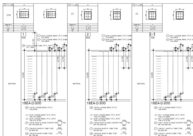
상세도
